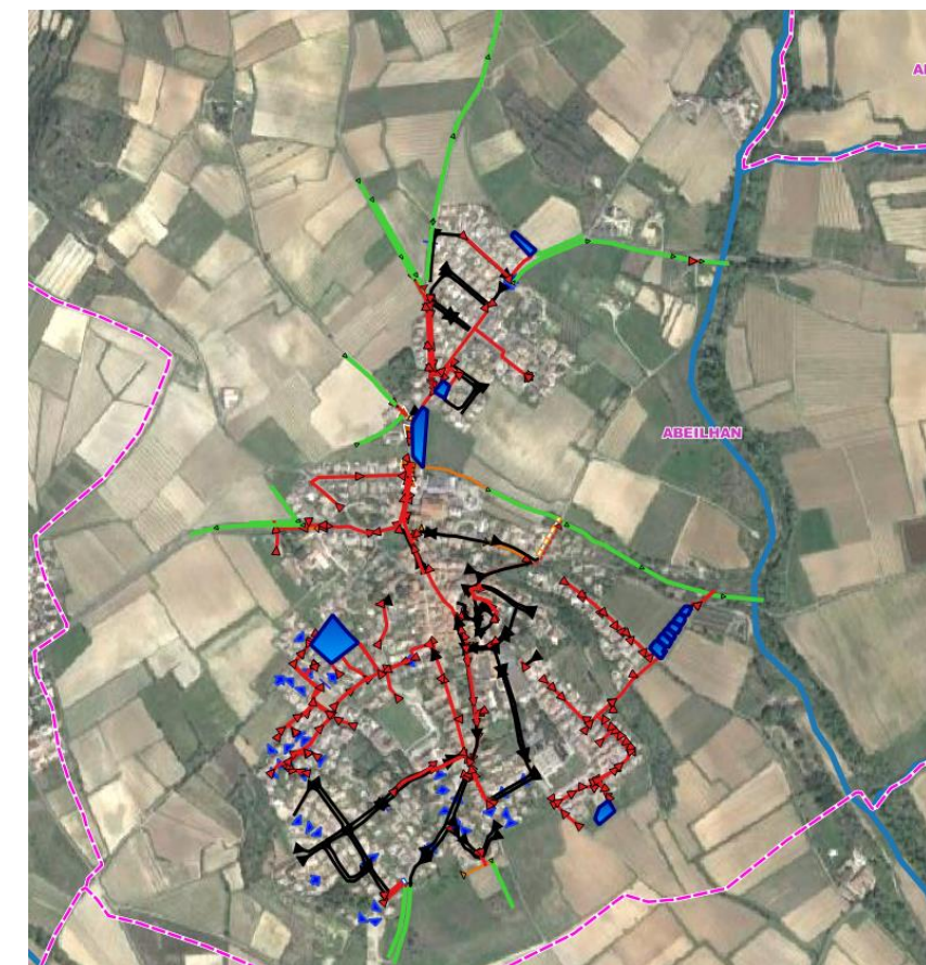
Architecture simplifiée du réseau d'eau pluviale sur la commune d'Abeilhan
