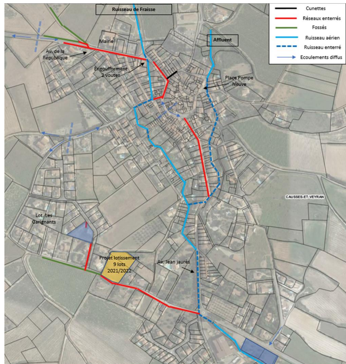
Figure 2 - Architecture simplifiée du réseau pluvial de la commune de Causses et Veyran
