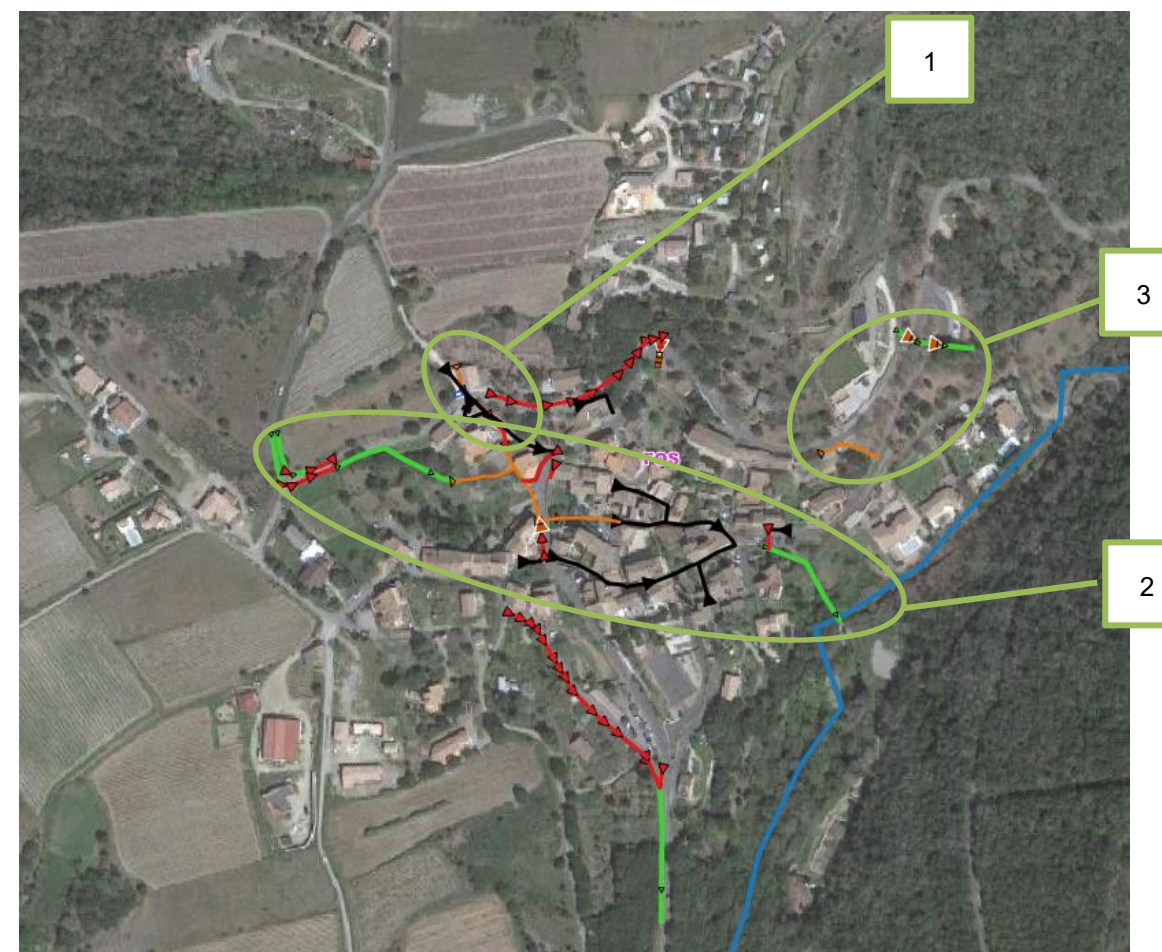
Figure 1 : Architecture simplifiée du réseau pluvial de la commune de Fos
