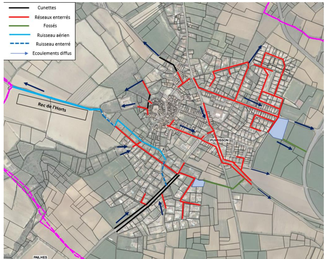
Figure 1 – Réseau pluvial simplifié de la commune de Puimisson
