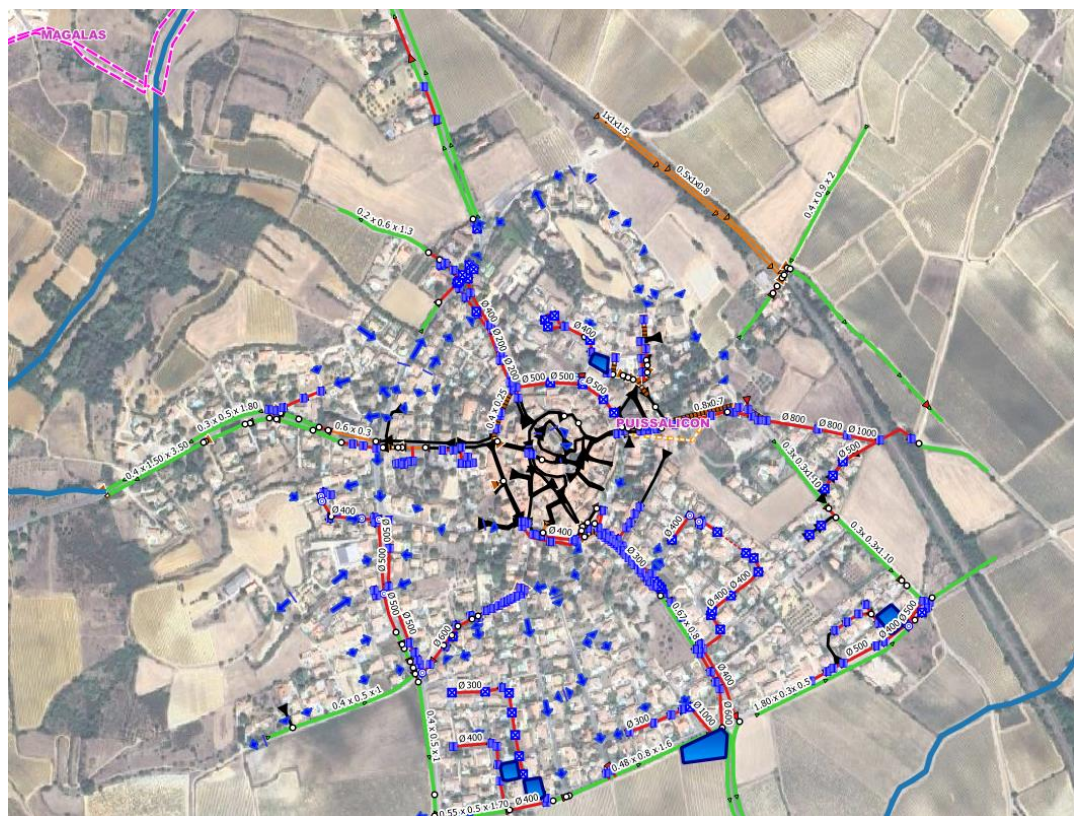
Figure 3 : Réseau pluvial de Puissalicon
