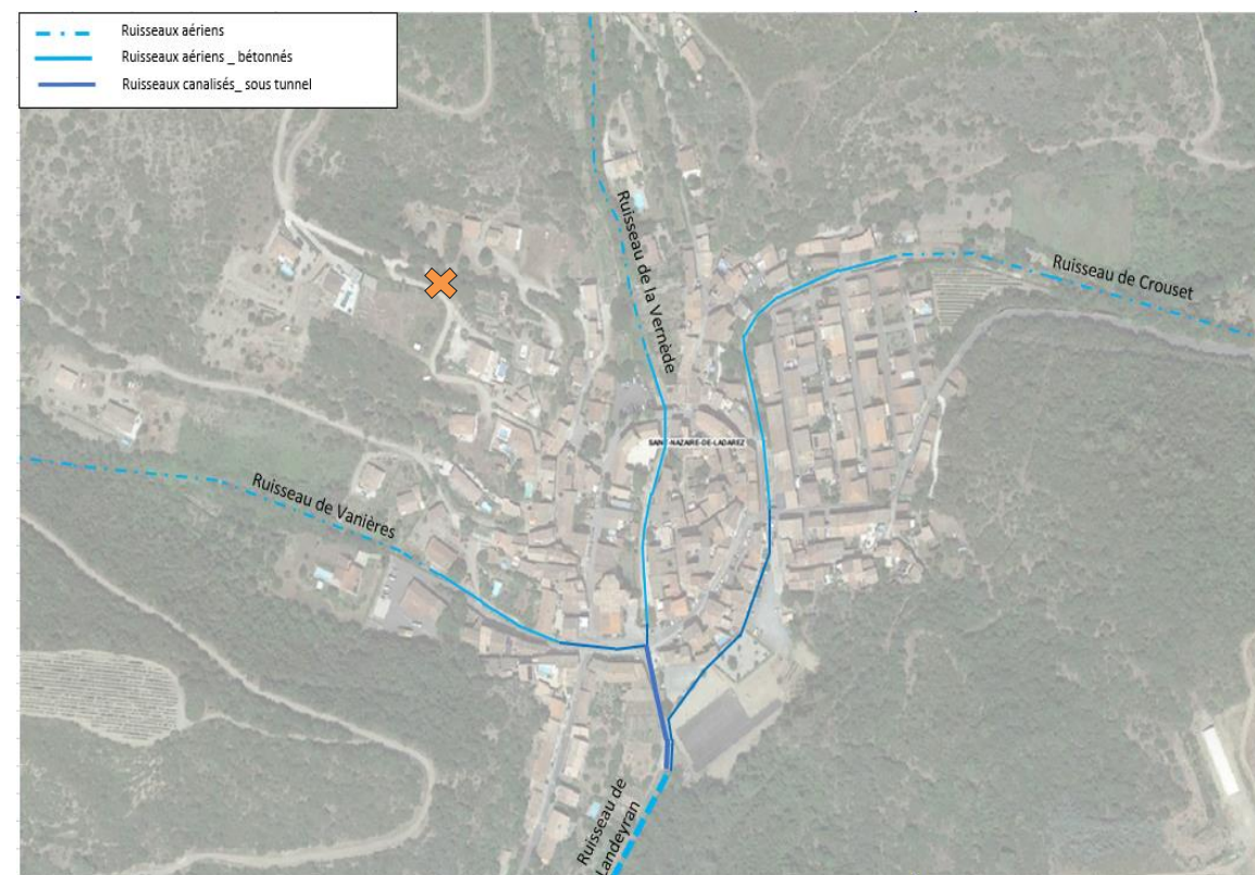
Architecture simplifiée du réseau d'eaux pluviales de la commune de Saint-Nazaire-de-Ladarez
