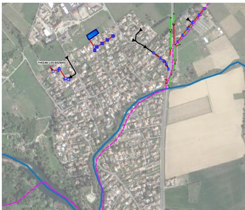
Figure 2 : Réseau d'eaux pluviales sur la commune de Thézan-lès-Béziers
