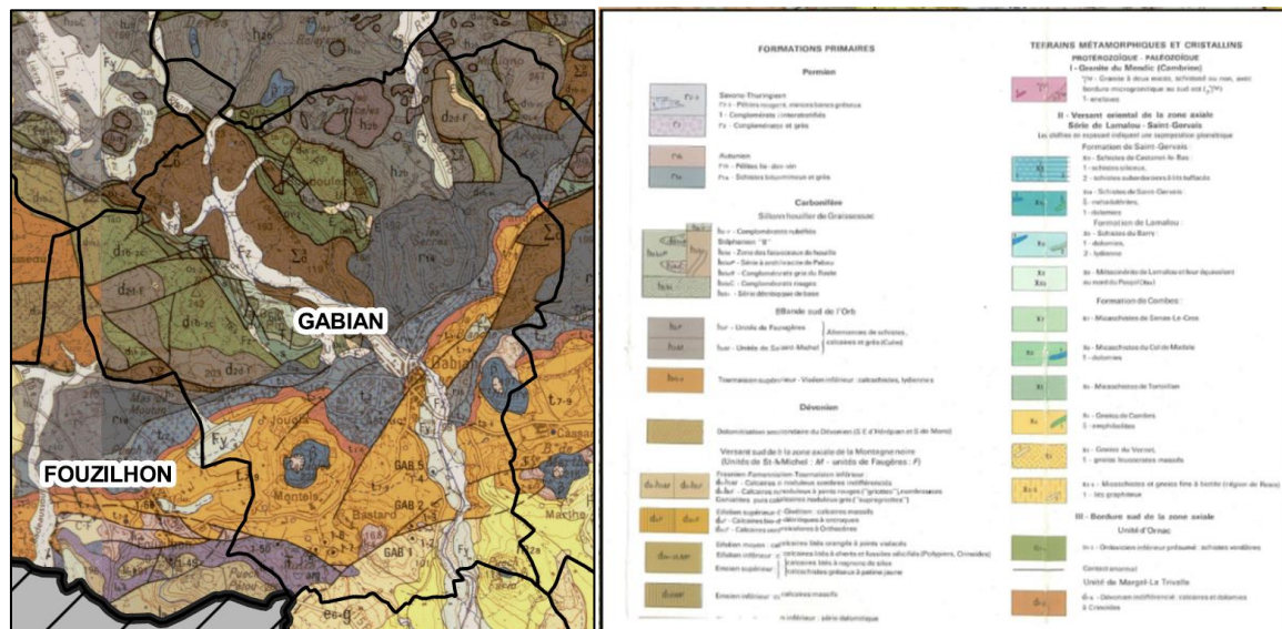
Figure 5: Contexte géologique sur la commune de Gabian
