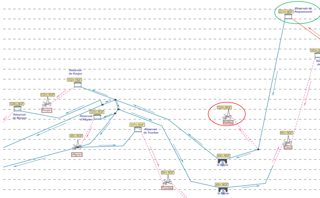
Figure 7: Synoptique de la rive droite du réseau d'eau potable du Syndicat Intercommunal des Eaux de la Vallée de l'Hérault vers la commune de Neffiès
