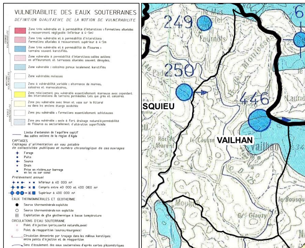
Figure 6: Contexte hydrogéologique de la commune de Vailhan
