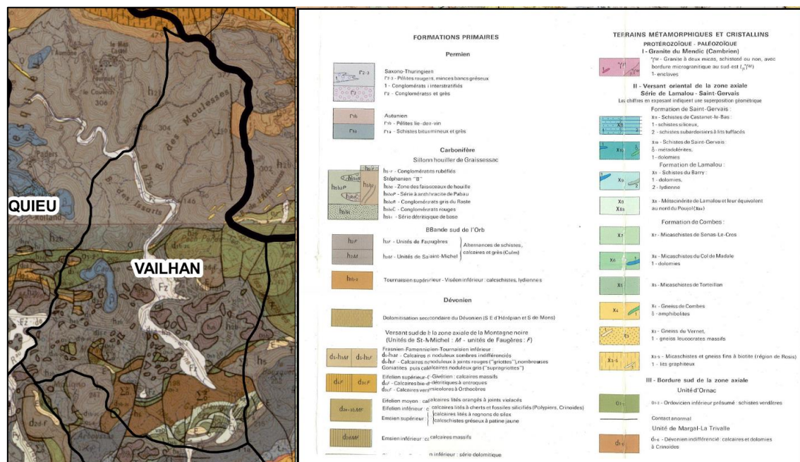
Figure 5: Contexte géologique sur la commune de Vailhan
