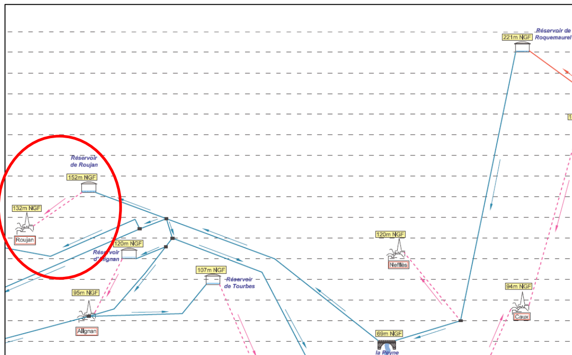
Figure 14 : Synoptique du fonctionnement du réseau
