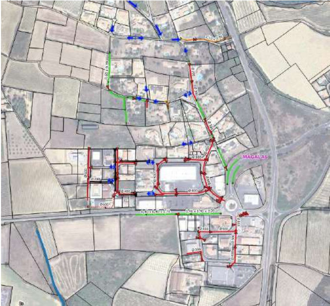
Figure 3 : Extrait du plan des réseaux pluviaux - secteur de la ZAE l'Audacieuce
